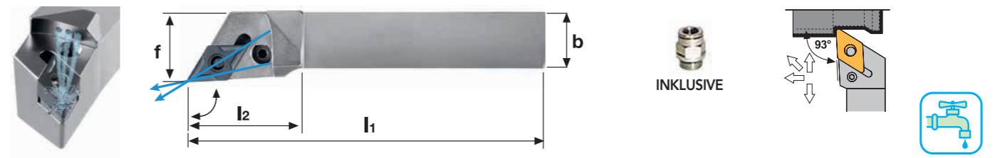
PDJNR/L Stahlschaft
