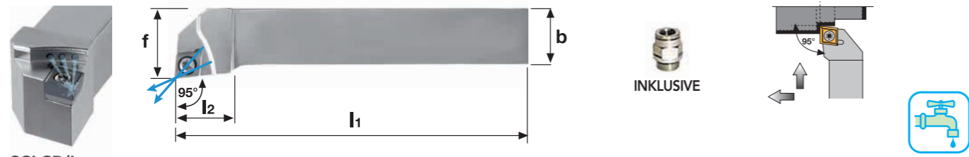
SCLCR/L Stahlschaft
