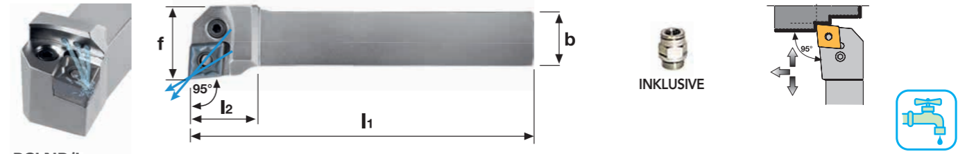
PCLNR/L Stahlschaft
