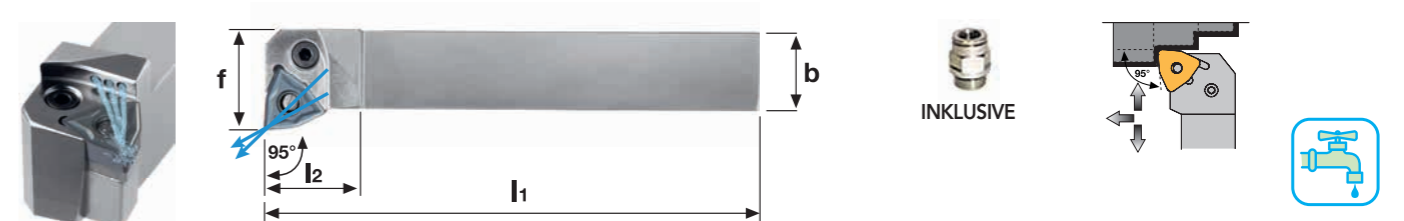
PWNLR/L Stahlschaft
