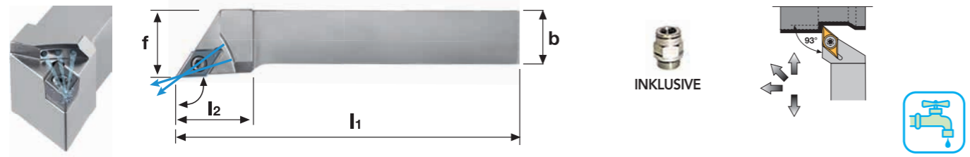
SDJCR/L Stahlschaft
