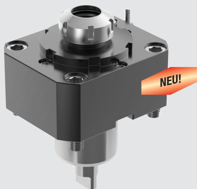
Angetriebene Spanneinheit • ER™
