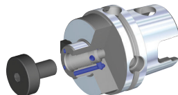
Aufsteckfräseraufnahmen
