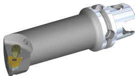
Schneidköpfe zur Innenbearbeitung
