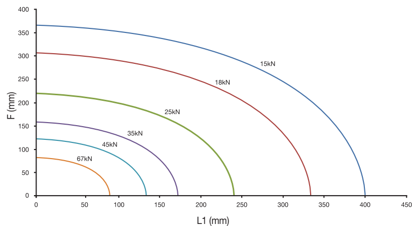
Maximale tangential Belastung für KM4X100
