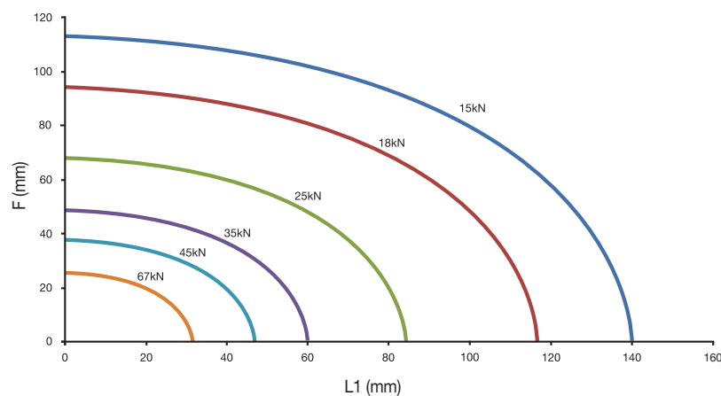
Maximale tangential Belastung für KM4X63
