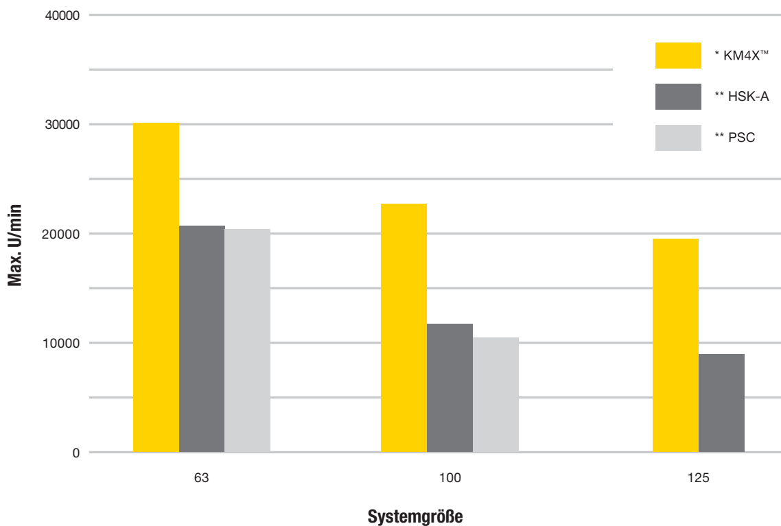
Maximal zulässige Drehzahlen U/min
