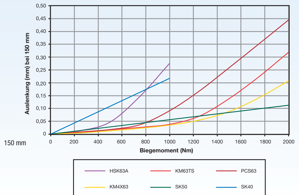
Diagramm zeigt den Biegesteifigkeitsvergleich von Steilkegel, HSK, PSC, KM-TS TM und KM4X TM .
