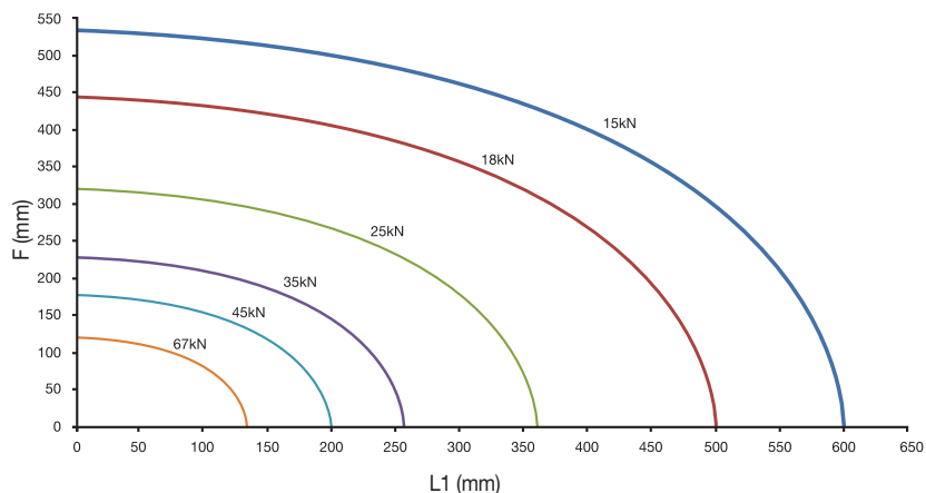
Maximale tangentielle Belastung für KM4X125
