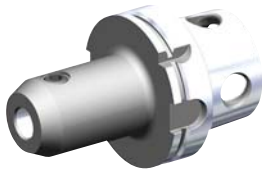
Whistle Notch Aufnahmen
