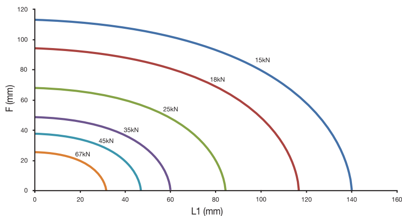
Maximale tangentielle Belastung für KM4X63
