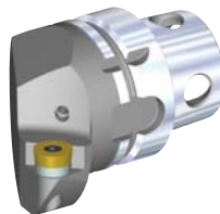
Schneidköpfe zum ISO Drehen
