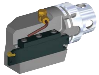
KM4X63 Schneidköpfe
