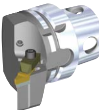
Schneidköpfe zum Top Notch™ Drehen
