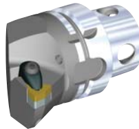
Kenclamp™ Schneidköpfe
